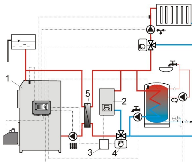
Hüdrauliline skeem täiendava katla avatud-suletud ahelas, milles 1 – juhtseade, 2 – lisakatel, 3 – vahereele, 4 – lülitusklapp (lõpplülititega), 5 – soojusvaheti, soovitatav seade: prioriteet KV = välja lülitatud, soojusvaheti = JAH.
